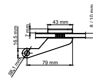
3-teiliges Band CREATIVO 3-part hinge CREATIVO
